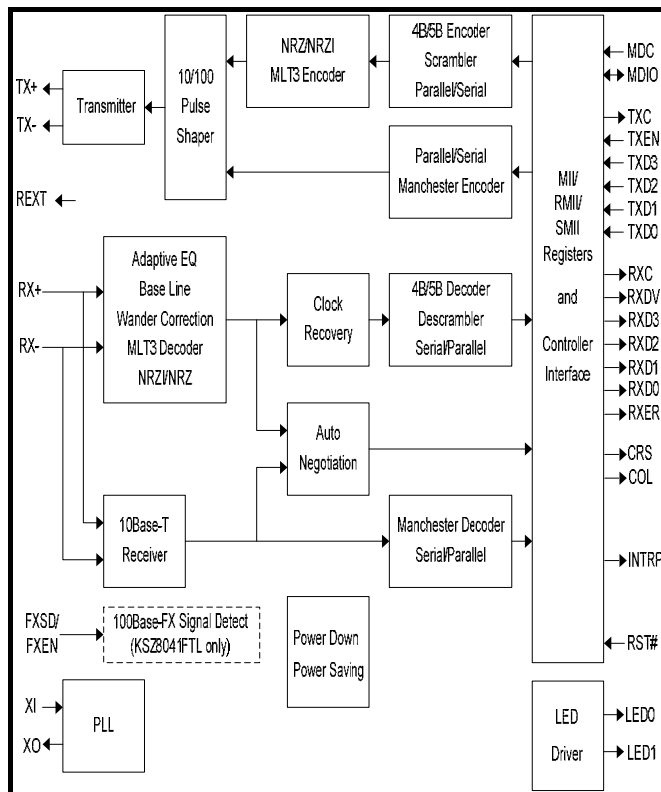
KSZ8041TL/FTL
