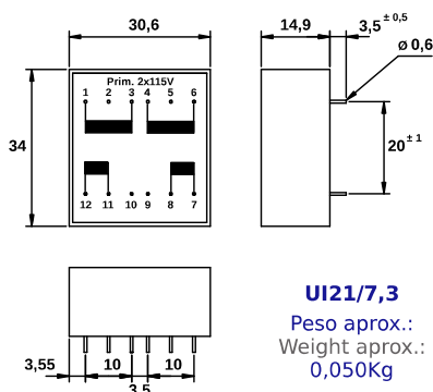
Dimensiones (mm) Dimensions (mm)
