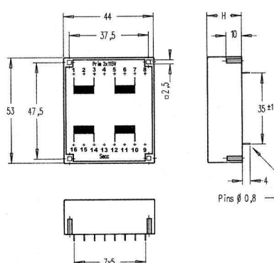
Dimensiones (mm) Dimensions (mm)
