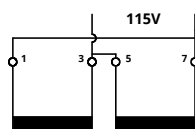
Conexión Paralelo 115V Parallel Connection 115V
